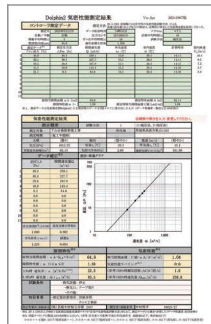
S様邸 気密性能測定結果
